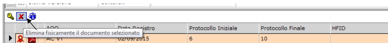
Fig. 14 – cancellazione documento
