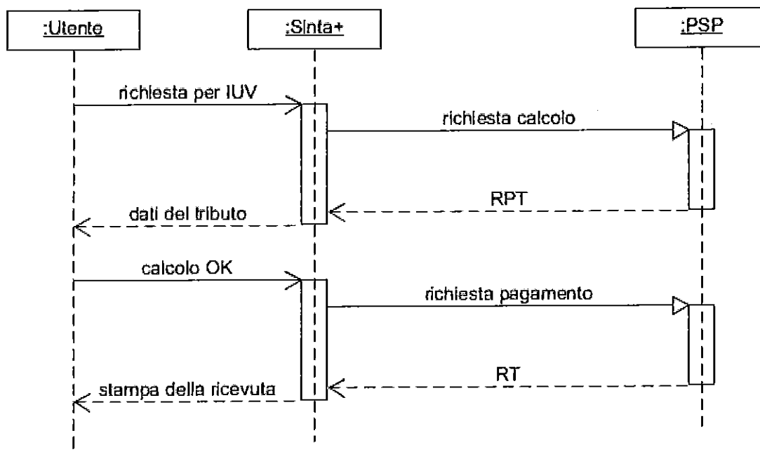
Figura 2. Sequence diagram di una richiesta di calcolo e pagamento di un tributo
