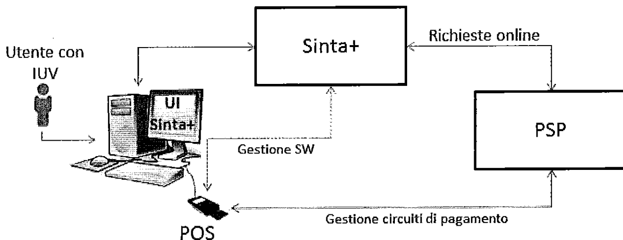
Figura 1. Schema interazioni online tra Sinta+ ed il PSP
