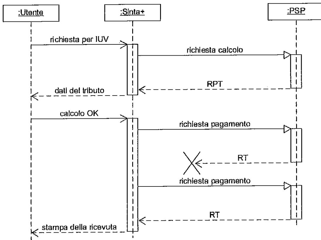
Figura 3. Sequence diagram di una richiesta di calcolo e pagamento con RT smarrita
