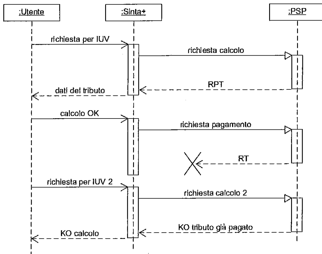
Figura 4. Sequence diagram di una richiesta di calcolo e pagamento con RT smarrita e nuova richiesta calcolo rifiutata
