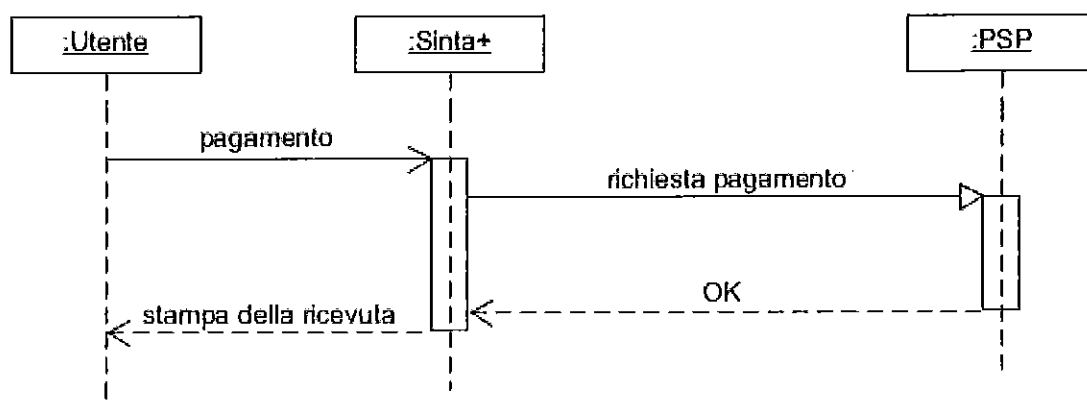
Figura 5. Sequence diagram di una richiesta di pagamento non legata ad un calcolo
